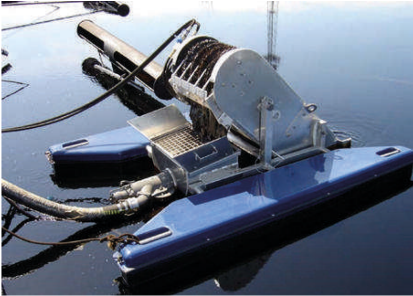
щёточный конвейерный нефтесборщик brush-type oil collector колектор нафтних деривата са четком
